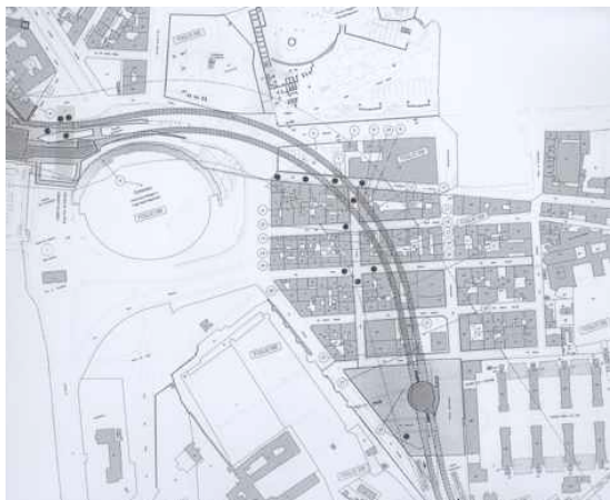
Il percorso delle due gallerie nel rione Celio
